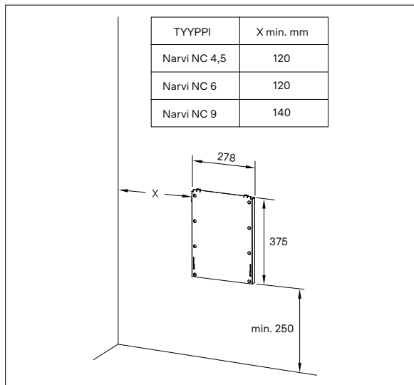
Kuva 6.9-1. Seinäkiinnityslevyn asennus.
