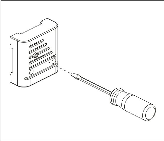
Kuva 7.12-1 Yllilämpösuojan uudelleenaktivointi
