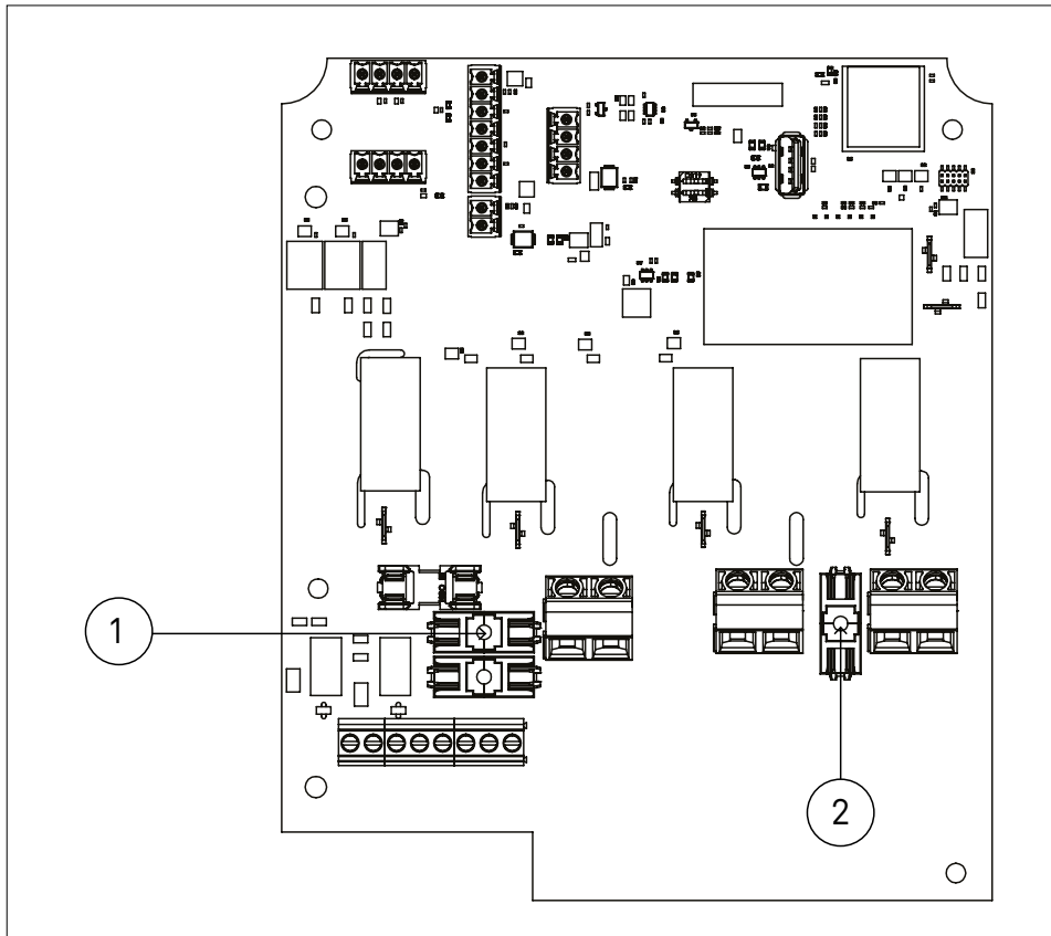
Bild 5.3-3. Kretskortets rörsäkringar
