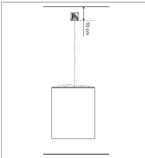
Kuva 6.5-1. Lämpötila-anturin asennus
