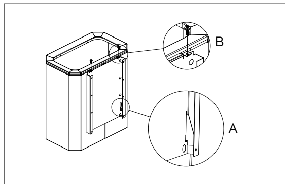
Kuva 6.9-2. kiukaan kiinnitys seinäkiinnityslevyyn
