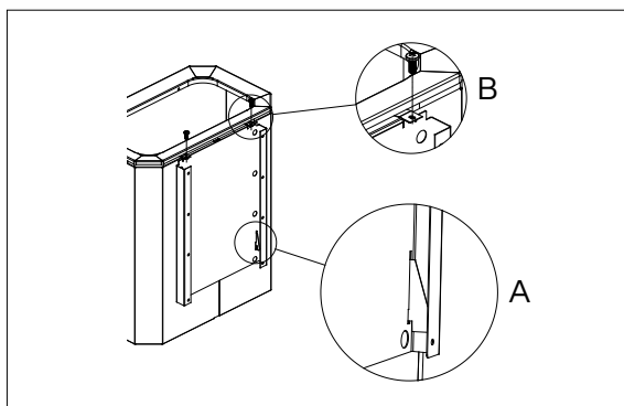
Bild 6.9-2. Aggregatets fastsättning i väggfästet
