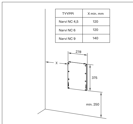
Bild 6.9-1. Installation av väggfästet
