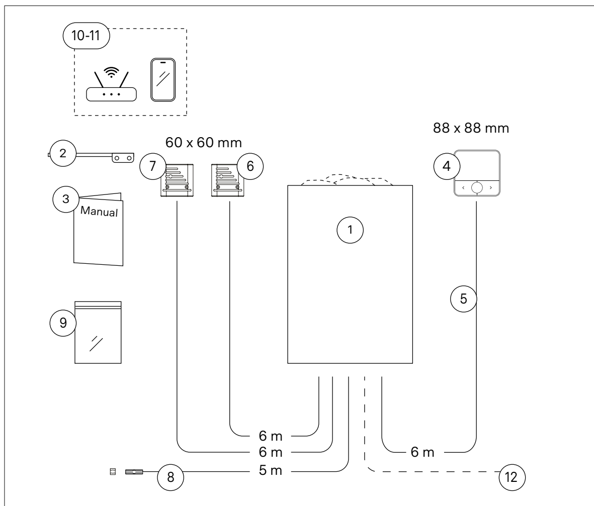
Bild 5.1-1. Bastusystemets delar
