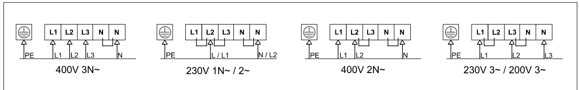
Bild 5.3-2. Kopplingschema för E-modell / med Flow-effektenhet
