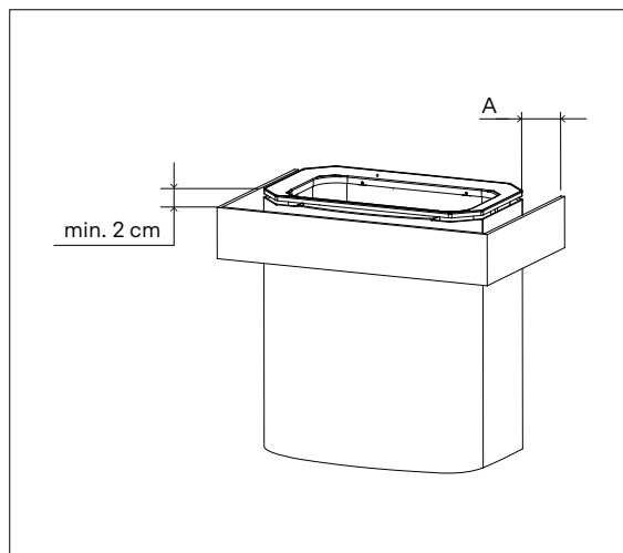
Bild 4.1-1. Aggregatets skyddsräcke
