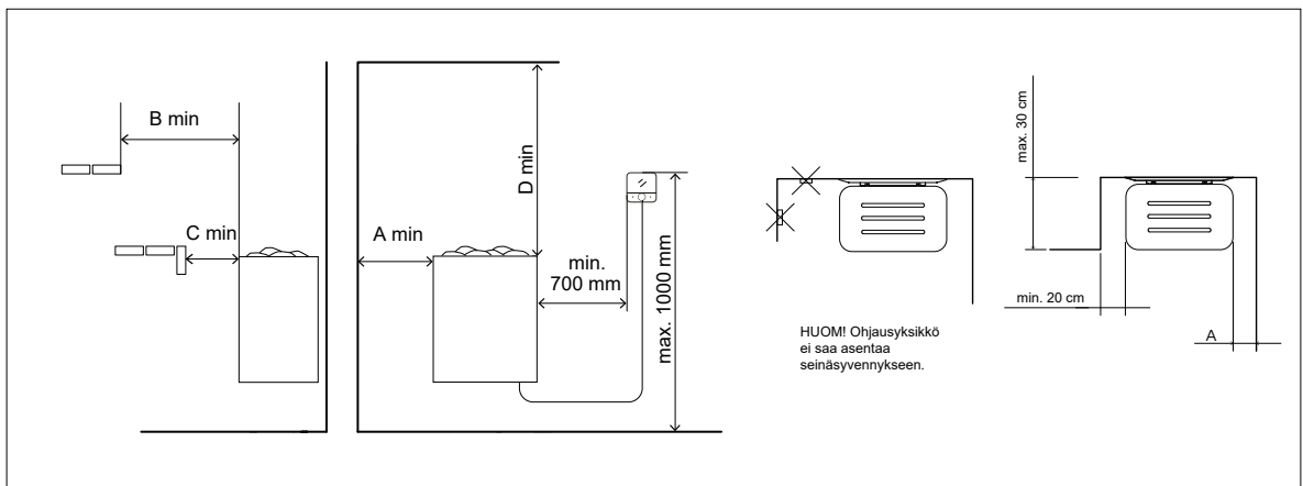
Kuva 6.1-1. Järjestelmän vähimmäisuojaetäisyydet
