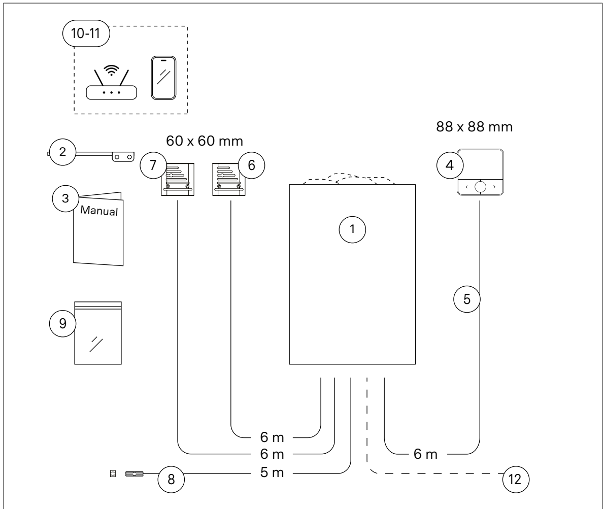
Kuva 5.1-1. Järjestelmän osat
