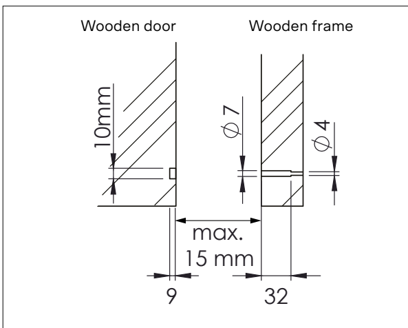
Abbildung 6.7-3. die Einbettung des Türsensors und des Magneten
