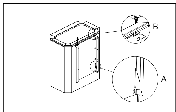
Abbildung 6.9-2. Befestigung des Saunaofens an der Wandmontageplatte
