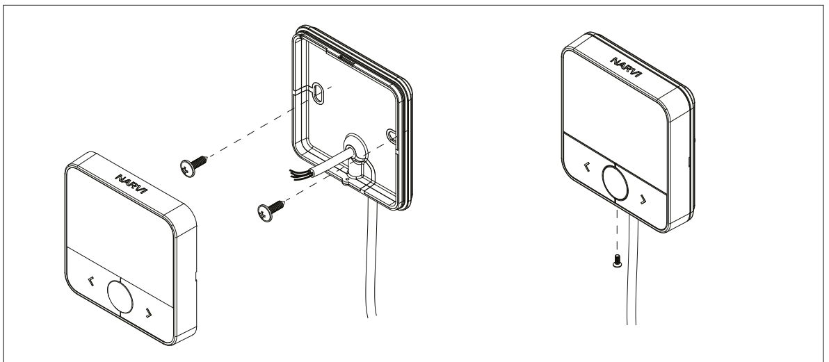
Kuva 6.4-1. Ohjainkotelon asennus
