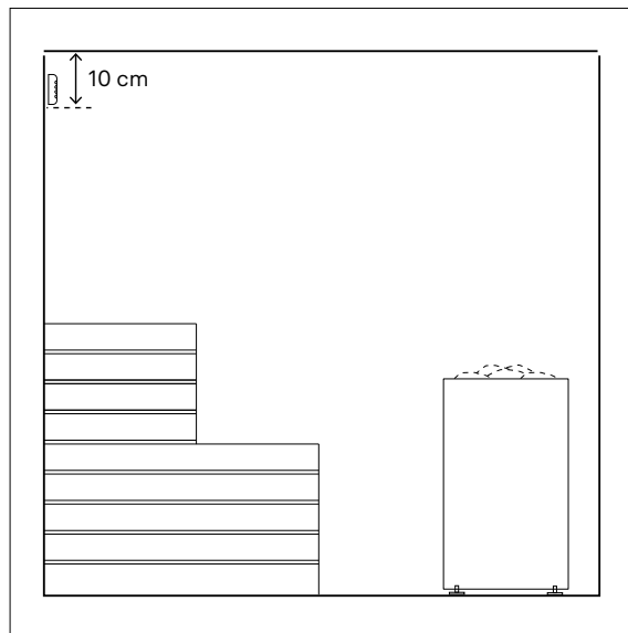
6.6-1. Installation av en fuktighetssensor
