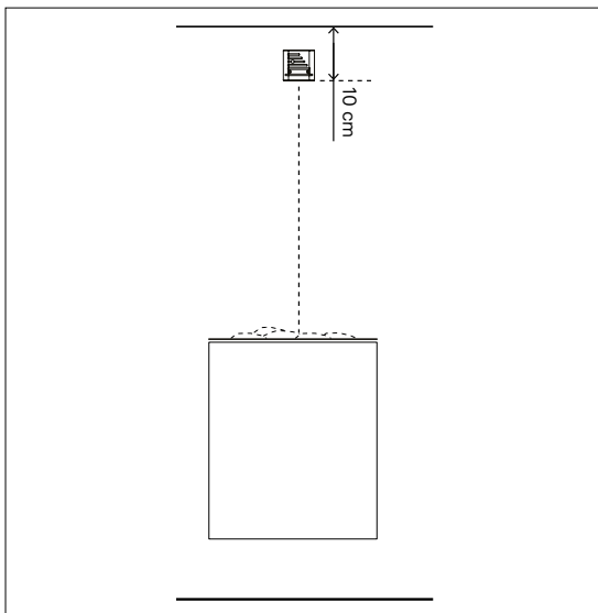
Bild 6.5-1. Installation av temperatursensorn
