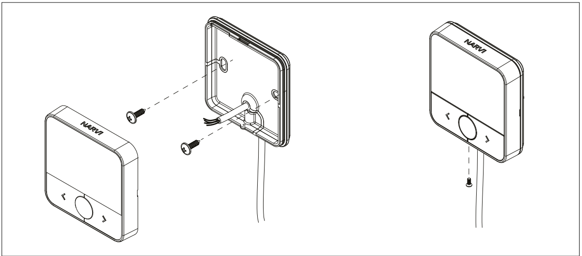
Abbildung 6.4-1. Installation des Gehäuses des Bedienfeldes
