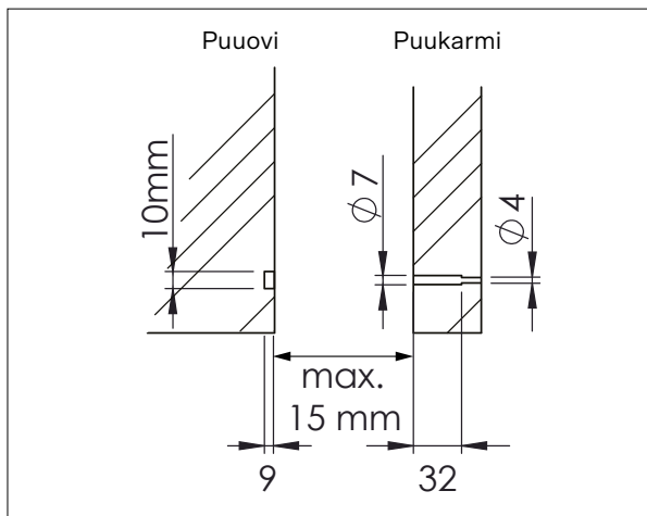
6.7-3. Ovikytkimen ja magneetin upotus
