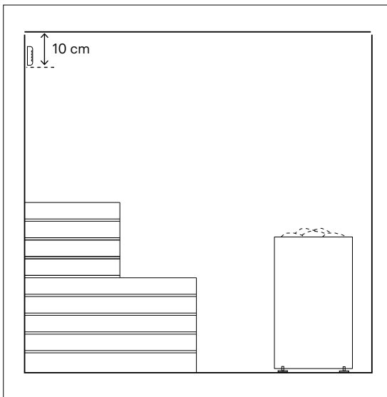
Kuva 6.6-1. Kosteusanturin asennus
