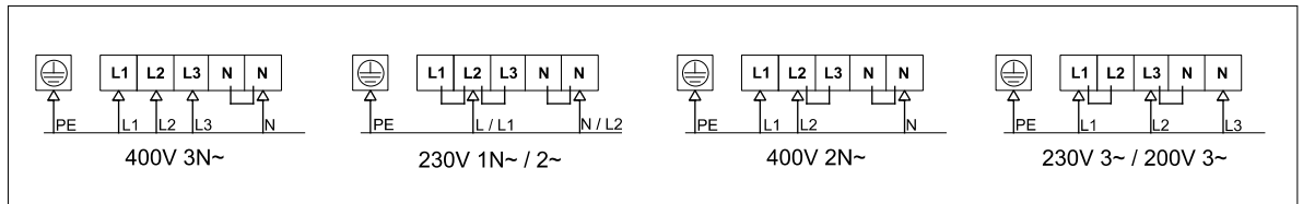
Abbildung 5.3-2. Schaltplan für das E-Modell / mit Flow-Leistungserweiterung
