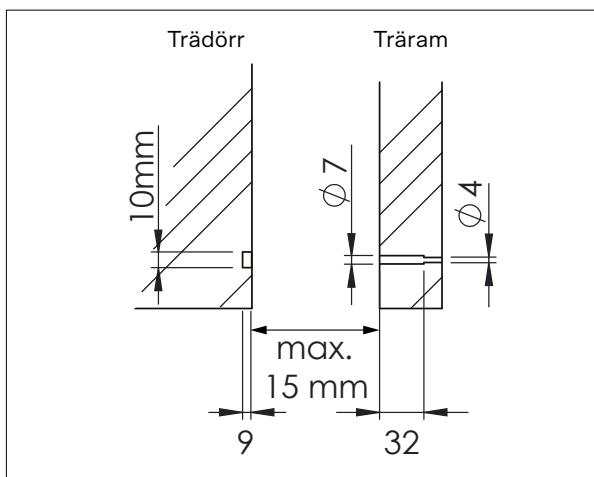
Bild 6.7-3. Infällning av dörrkontakt och magnet
