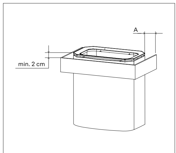
Abbildung 4.1-1. Schutzgeländer für den Saunaofen
