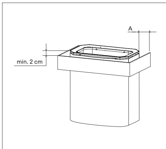
Kuva 4.1-1. Kiukaan suojakaide
