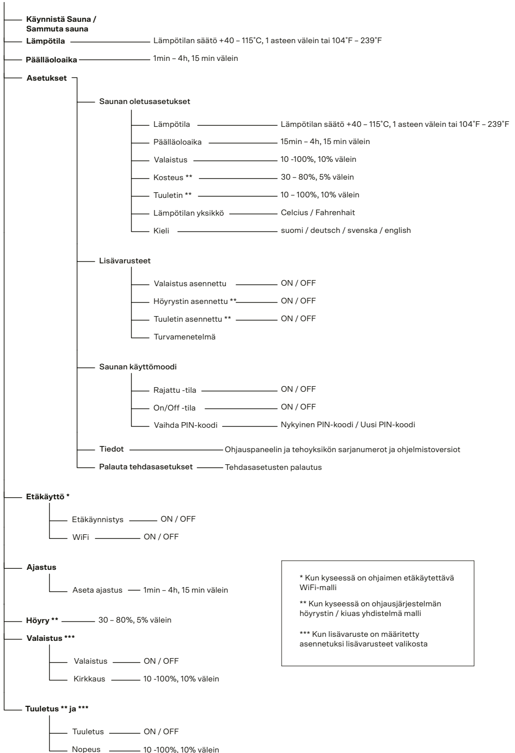
Taulukko 7.1-1. Käyttöliittymäkaavio
