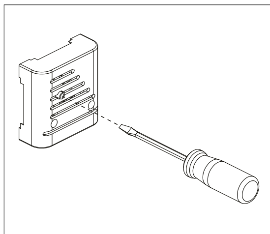
Kuva 7.12-1. Yllilämpösuojan uudelleenaktivointi
