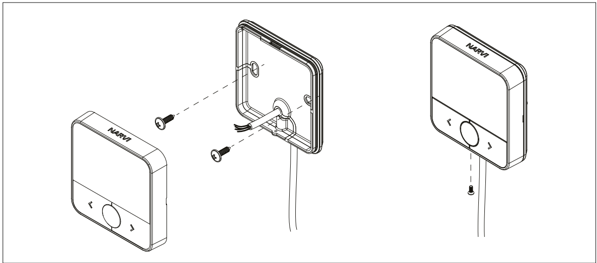
Kuva 6.4-1. Ohjainkotelon kiinnitys seinään ja kotelon kiinnitys
