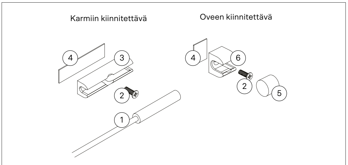
Kuva 6.7-1. Ovikytkinsarja: 1) Ovikytkin liitäntäkaapelilla, 2) Ruuvi 3) Karmin kytkinpidike 4) Tarra 5) Magneetti 6) Oven magneettipidike
