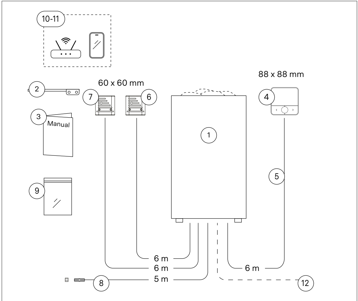
Kuva 5.1-1. Järjestelmän osat
