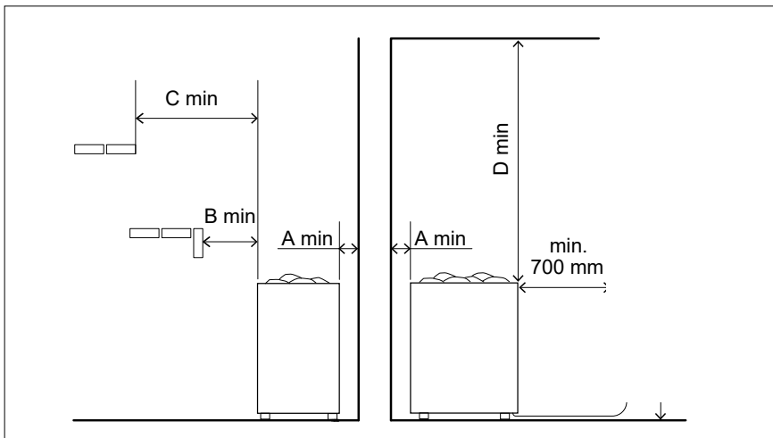
Kuva 6.1-1. Järjestelmän vähimmäissuojaetäisyydet
