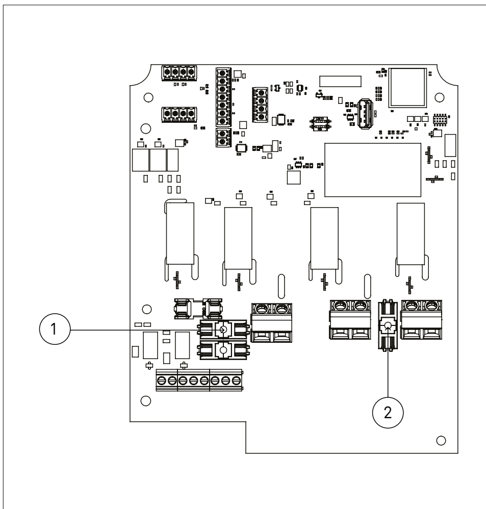
Abbildung 5.3-2. Sicherungen für Leiterplatten
