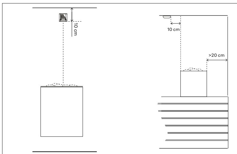
Abbildung 6.5-1. Installation des Temperatursensors
