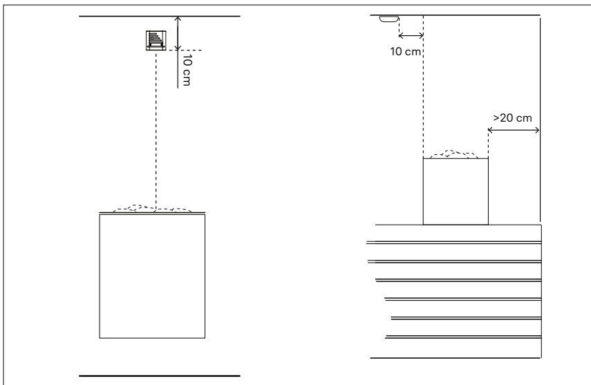
Kuva 6.5-1. Lämpötila-anturin asennus
