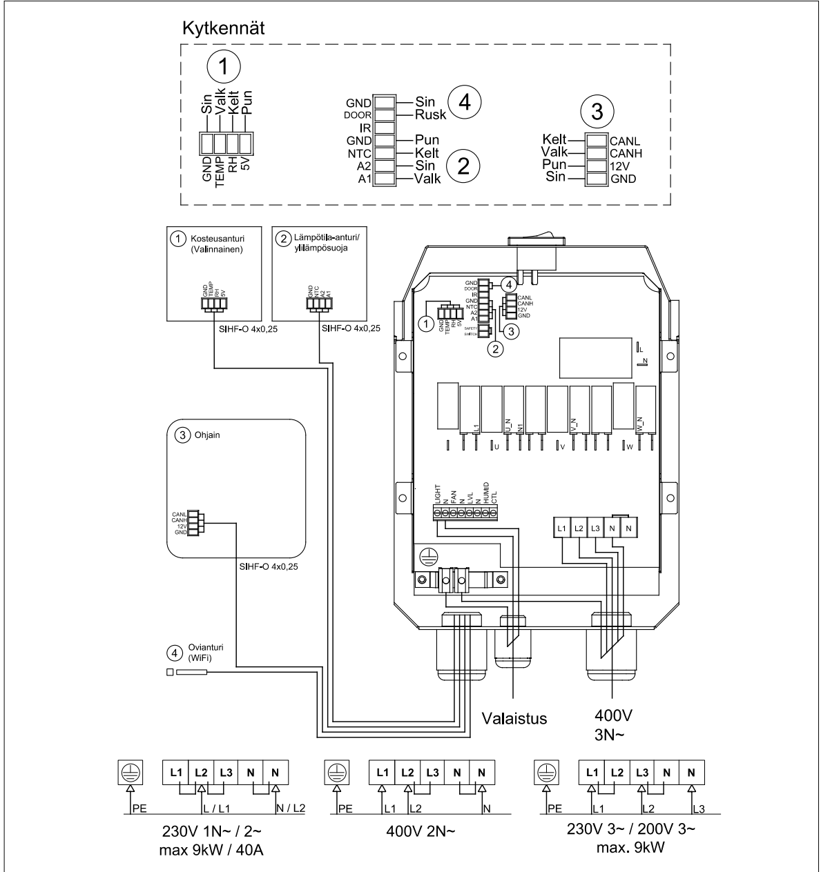
Kuva 5.3-1. Kytkentäkaavio
