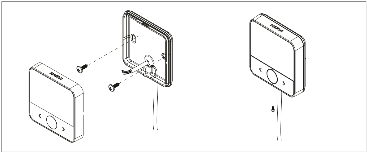
Abbildung 6.4-1. Installation des Gehäuses des Bedienfeldes
