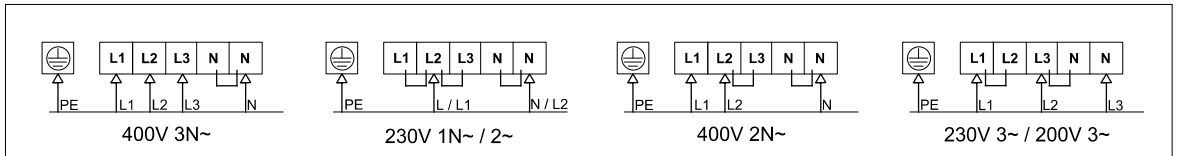
Kuva 5.3-2. KytKentäkaavio E-malli / Flow lisätehoyksiköllä
