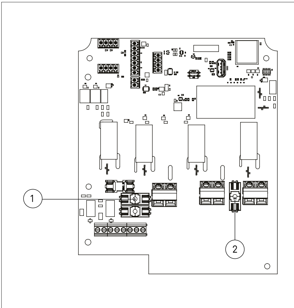
Kuva 5.3-2. Piirikortin lasiputkisulakkeet
