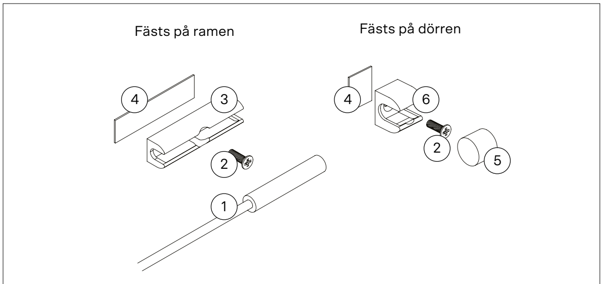
Bild 6.7-1. Dörrkontaktens uppsättning: 1) Dörrkontakt med anslutningskabel, 2) Skruv 3) Fäste för dörramen 4) Klistermärke 5) Magnet 6) Magnetfäste för dörren
