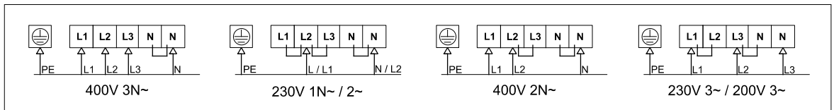
Abbildung 5.3-2: Verbindungsdiagramm E-Modell / Flow mit zusätzlicher Leistungseinheit
