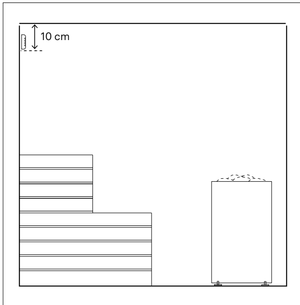
Kuva 6.6-1. Kosteusanturin asennus
