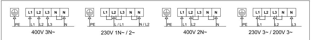
Bild 5.3-2. Kopplingschema E-modell / Flow med extra effektenhet
