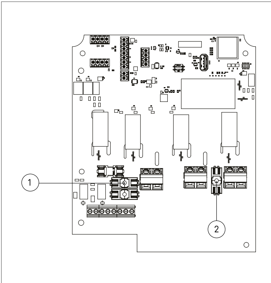
Bild 5.3-2. Kretskortets glasrörssäkringar
