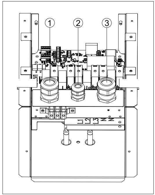
Kuva 6.3-1. Kytkentäkotelon läpviennit
