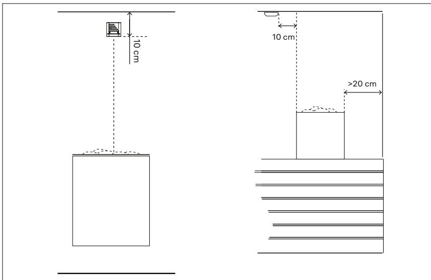
Bild 6.5-1. Installation av temperatursensorn
