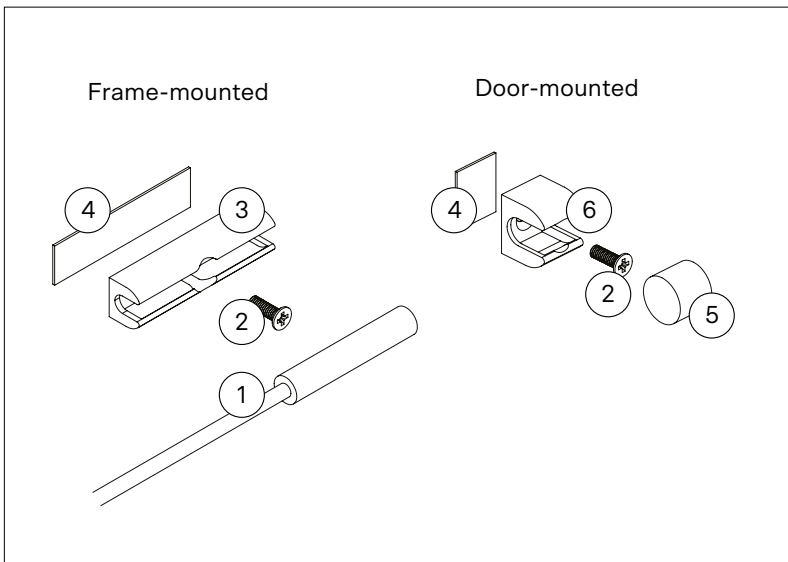
Abbildung 6.7-1. Türsensor einstellen: 1) Türsensor mit Anschlusskabel 2) Schraube 3) Rahmenschalterhalter 4) Aufkleber 5) Magnet 6) Türmagnethalter
