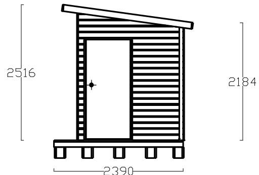
JULKISIVU VASEMMALTA
