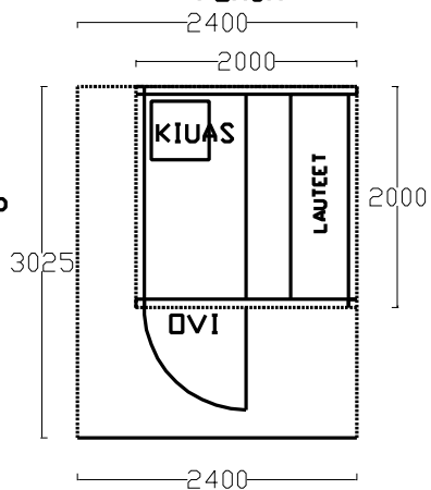
POHJA
