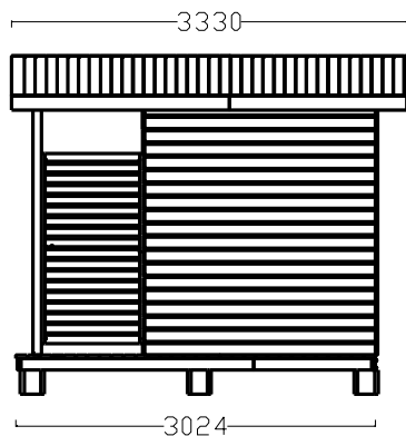
JULKISIVU EDESTÄ
