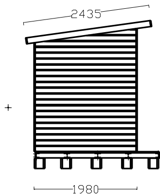
JULKISIVU VASEMMALTA
